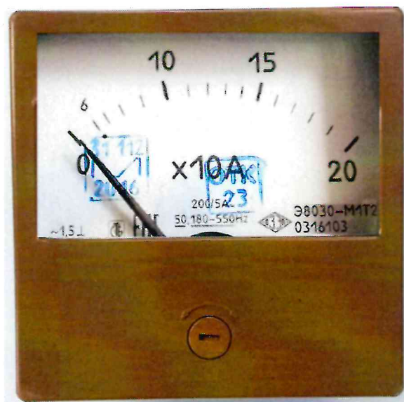
Рисунок 2 - Общий вид амперметров Э8030-М1Т2 тропического исполнения
