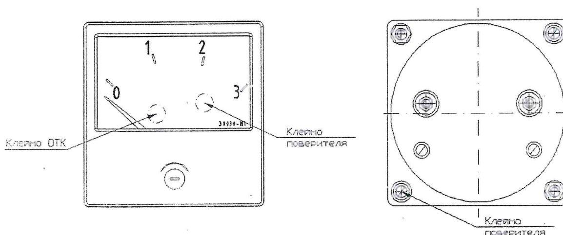
Рисунок 4 – Схема клеймения амперметров Э8030-М1
