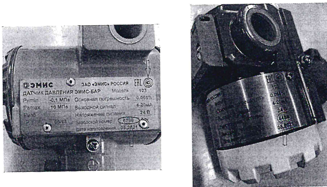
Рисунок 2 – Места расположения заводского номера и знака утверждения типа
