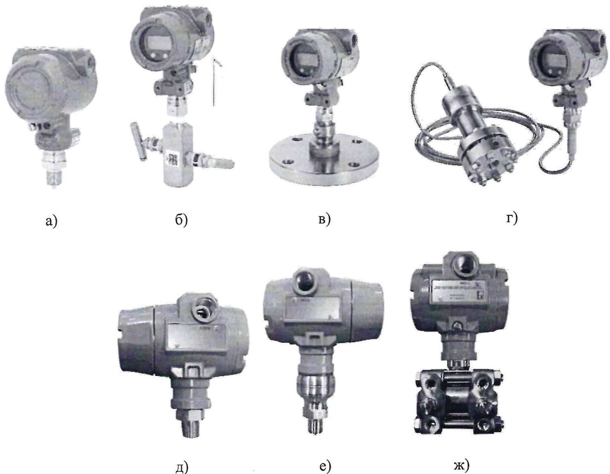
Рисунок 1 – Общий вид датчиков давления Метран-75 а), д), е) - датчики штуцерного исполнения; б) датчик в сборе с клапанным блоком; в) датчик в сборе с выносной разделительной мембраной прямого монтажа; г) датчик в сборе с выносной разделительной мембраной, соединенной капилляром, ж) датчик фланцевого исполнения
