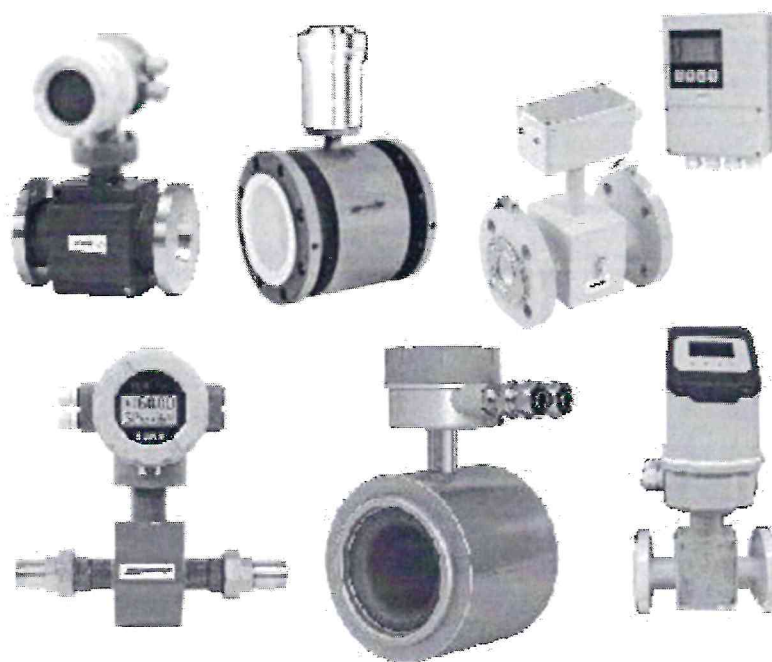
Рисунок 1 – Общий вид расходомеров-счетчиков электромагнитных Энергия-Э
