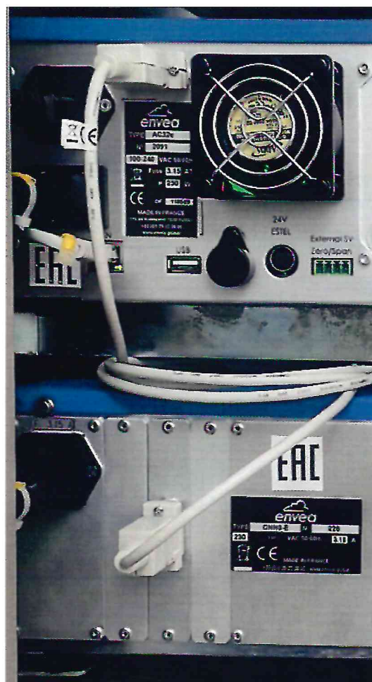
Рисунок 1.2 – Фотография маркировки газоанализатора AC32e № 2091 с преобразователем аммиака CNH3-E № 229
