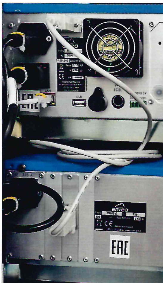
Рисунок 1.2 – Фотография маркировки газоанализатора AC32e № 2090 с преобразователем аммиака CNH3-E № 228
