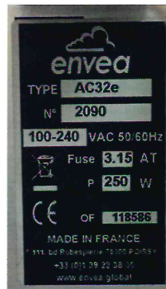
Рисунок 1.1 – Фотографии общего вида газоанализатора AC32e № 2090 с преобразователем аммиака CNH3-E № 228
