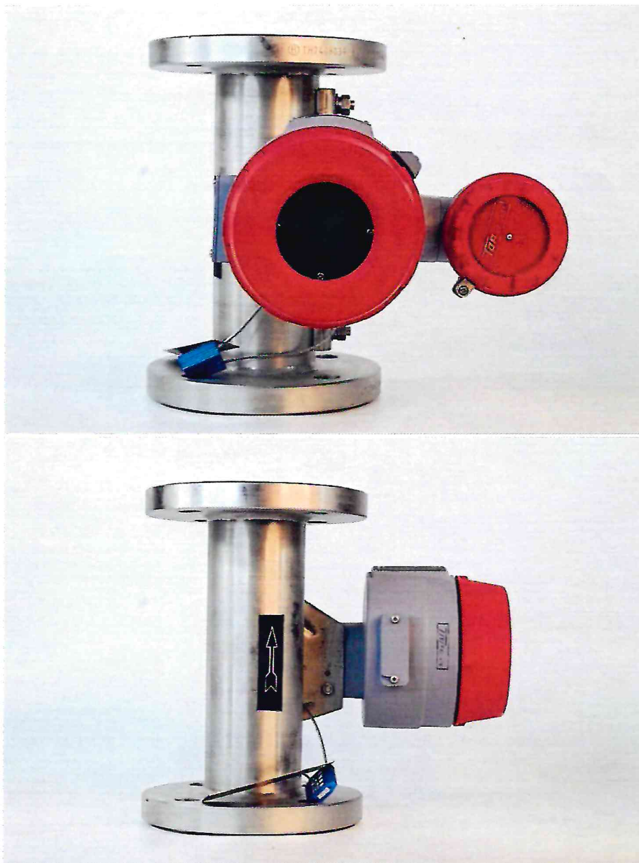
Рисунок 1.1 – Фотографии общего вида расходомера поплавкового MTF-B7W4/97iDC № 231008833 (изображение носит иллюстративный характер)
