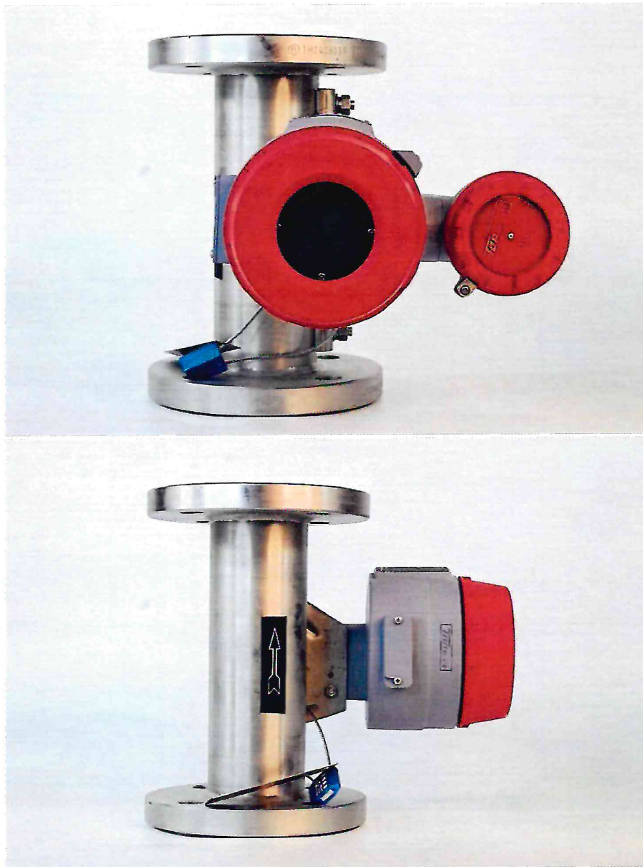
Рисунок 1.1 – Фотографии общего вида расходомера поплавкового MTF-B7W4/97iDC № 231008851 (изображение носит иллюстративный характер)
