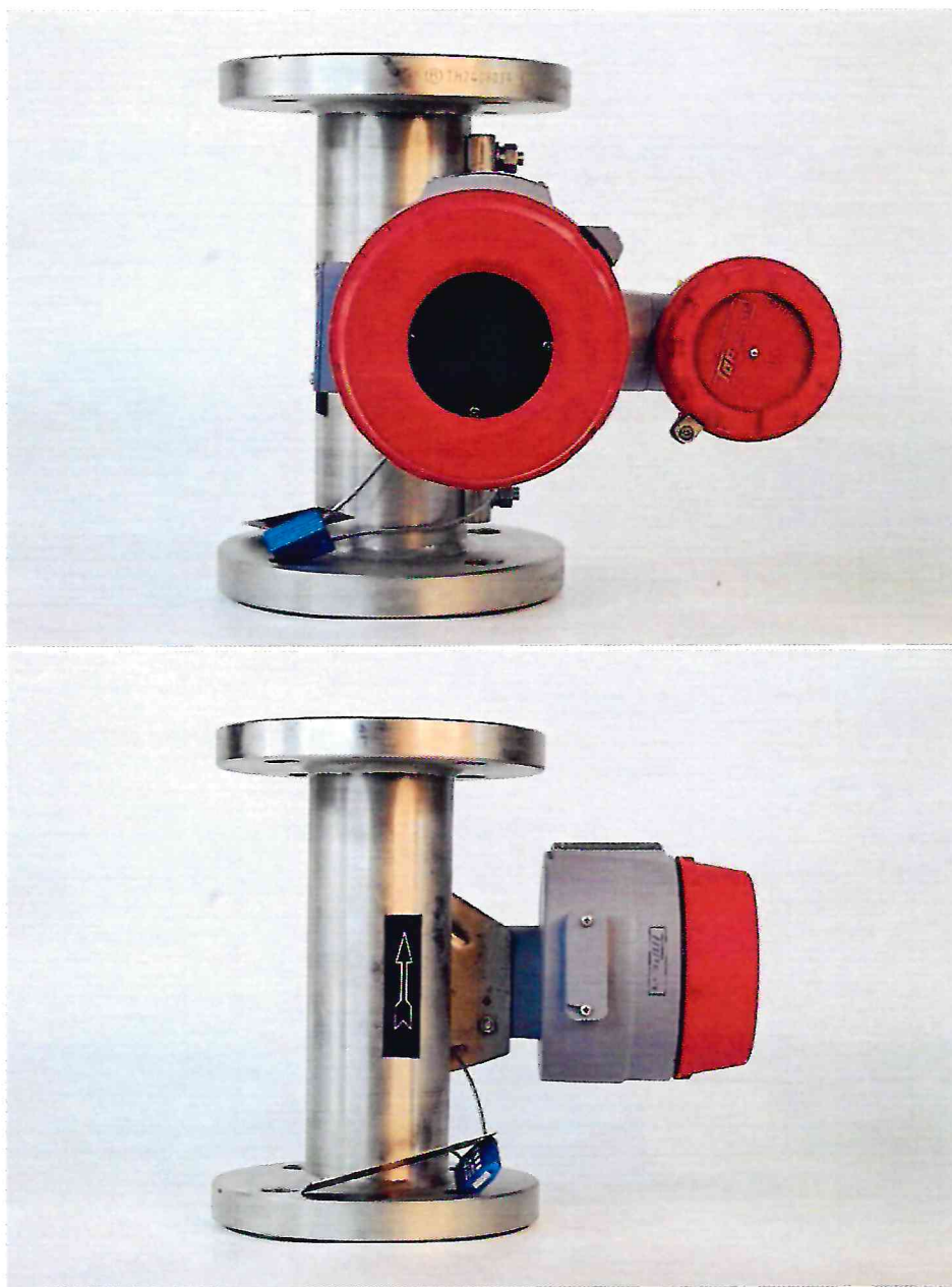
Рисунок 1.1 – Фотографии общего вида расходомера поплавкового MTF-B7W3/97iDC № 231008855 (изображение носит иллюстративный характер)
