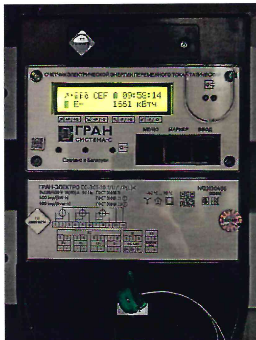
Измерительный канал № 4
