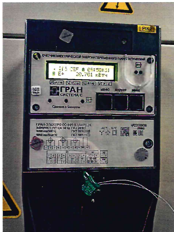
Измерительный канал № 2
