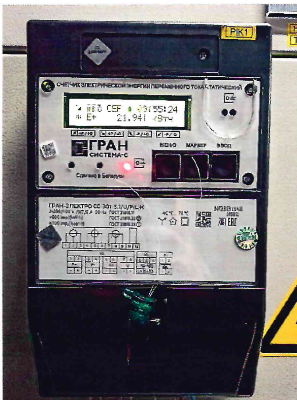
Измерительный канал № 1
