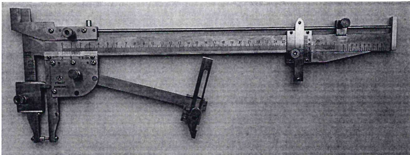
Рисунок 1 – Общий вид штангенциркулей путевых ПШВ-01
