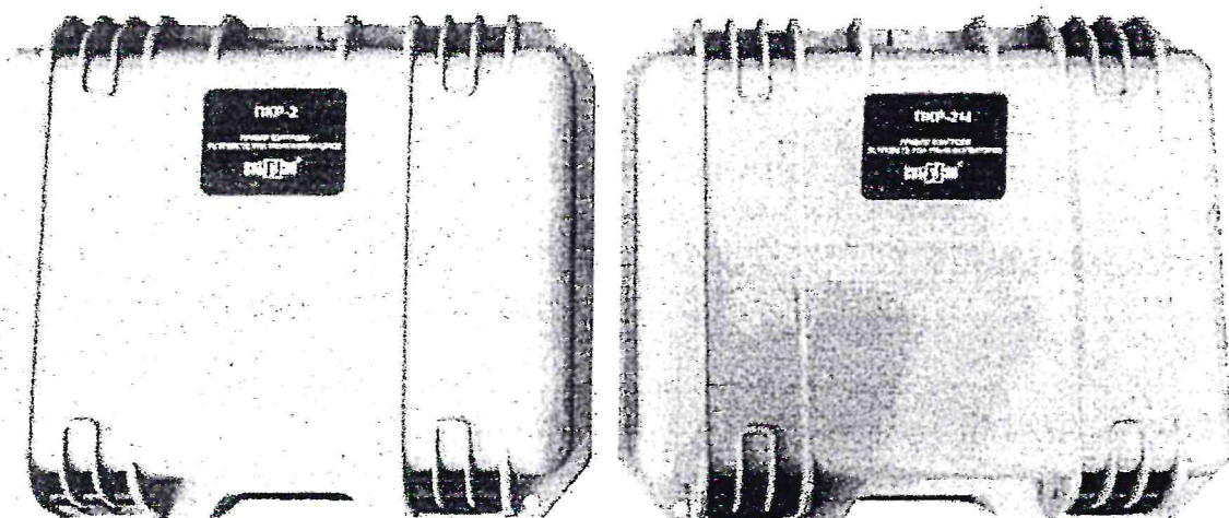
Рисунок 1 – Прибор ПКР-2 и его модификация ПКР-2М
