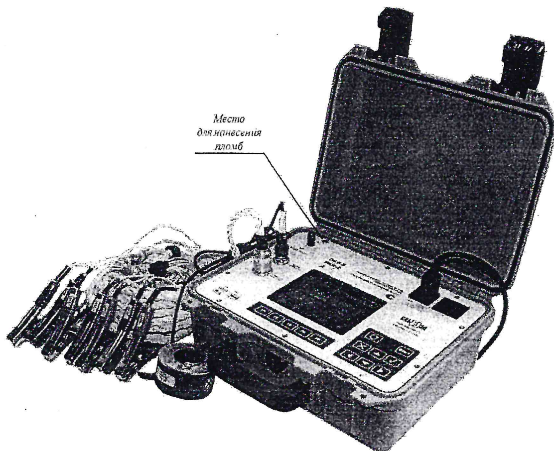
Рисунок 2 – Измерительный блок, датчик угловых перемещений, комплект монтажных приспособлений и комплект кабелей
