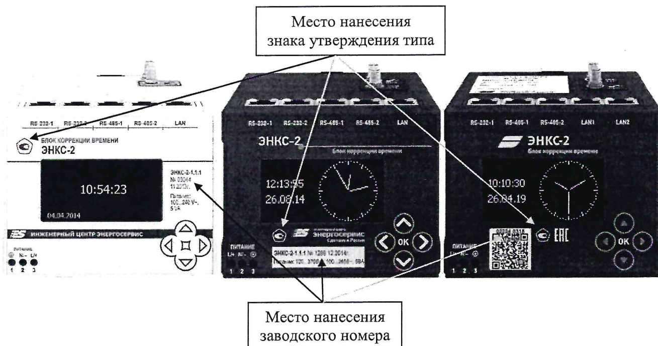
Рисунок 1 – Общий вид БКВ, места нанесения знака утверждения типа и заводского номера
