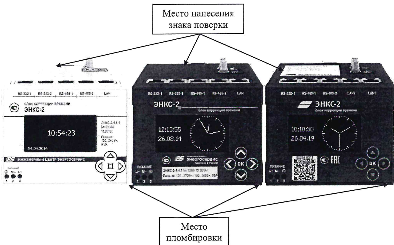
Рисунок 2 – Схема пломбировки от несанкционированного доступа, обозначение мест нанесения знака поверки
