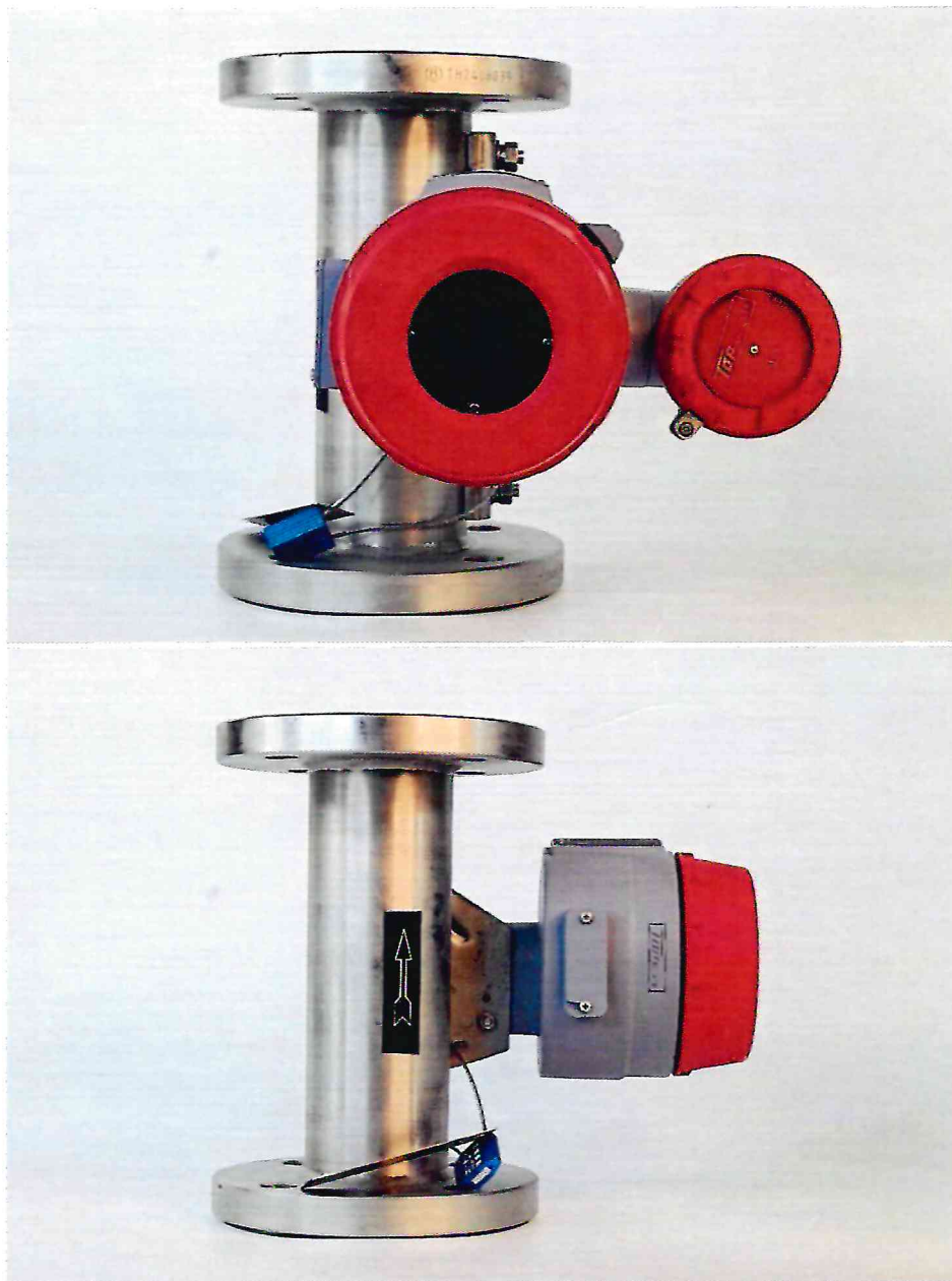
Рисунок 1.1 – Фотографии общего вида расходомера поплавкового МТФ-В6Z7/4iDC № 240706047 (изображение носит иллюстративный характер)
