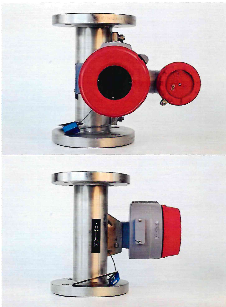
Рисунок 1.1 – Фотографии общего вида расходомера поплавкового МТF-B6W4/4iDC № 240706062 (изображение носит иллюстративный характер)
