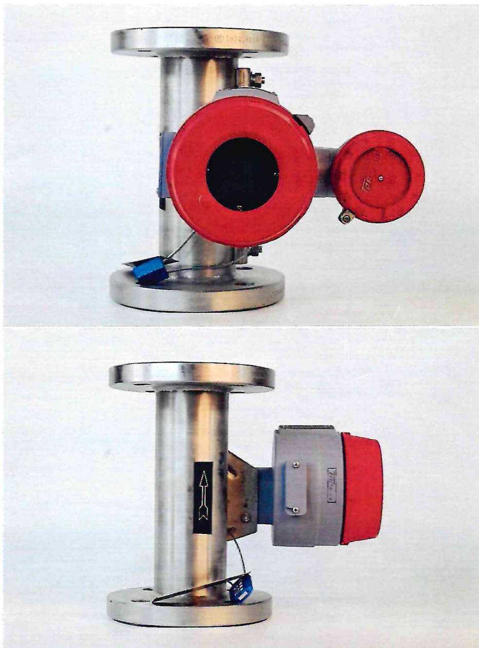
Рисунок 1.1 – Фотографии общего вида расходомера поплавкового МТФ-В6W4/4iDC № 240706058 (изображение носит иллюстративный характер)
