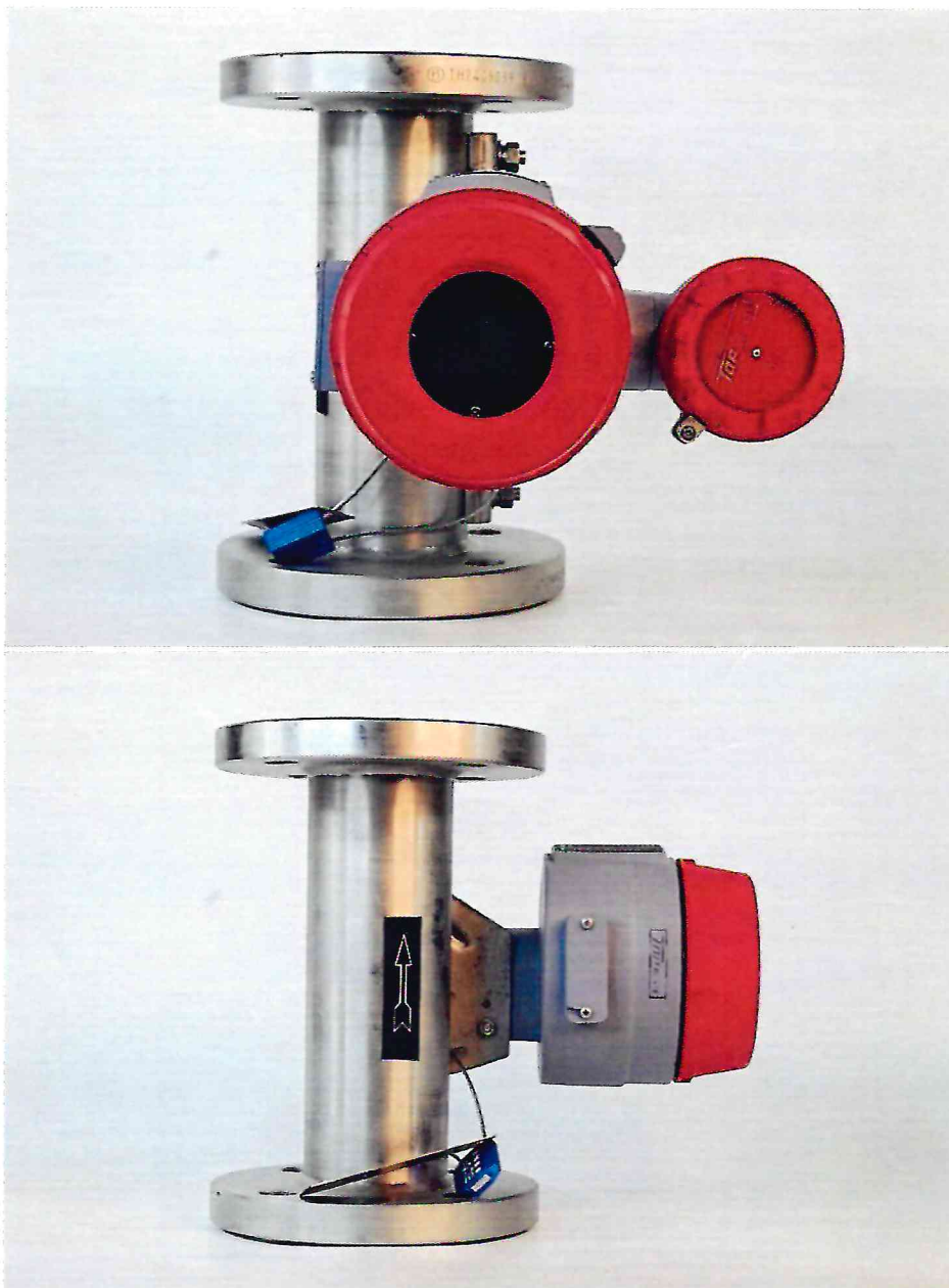
Рисунок 1.1 – Фотографии общего вида расходомера поплавкового МТF-B6W4/4iDC № 240706057 (изображение носит иллюстративный характер)
