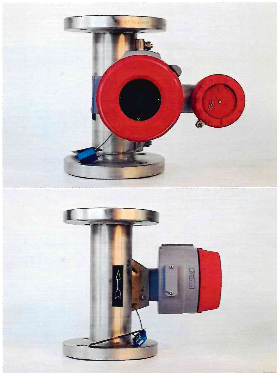
Рисунок 1.1 – Фотографии общего вида расходомера поплавкового МТФ-В6Z7/4iDC №240706053 (изображение носит иллюстративный характер)
