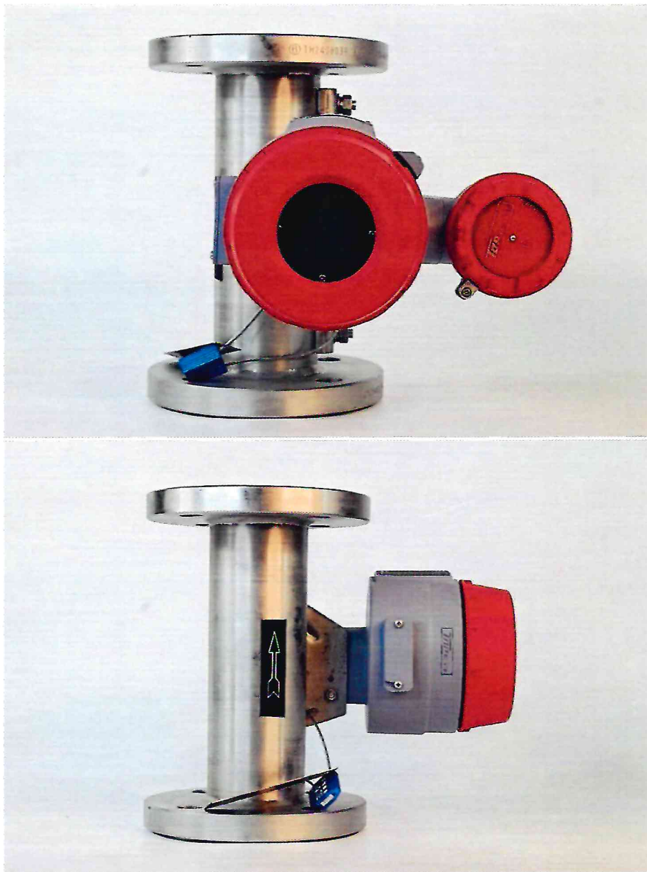
Рисунок 1.1 – Фотографии общего вида расходомера поплавкового МТФ-В6Z7/4iDC №240706048 (изображение носит иллюстративный характер)
