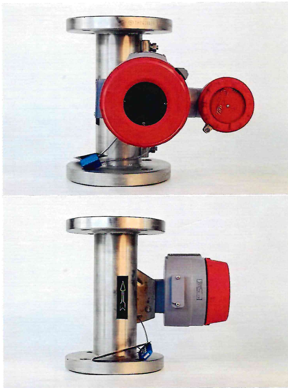
Рисунок 1.1 – Фотографии общего вида расходомера поплавкового MTF-B6Z7/4iDC №240706052 (изображение носит иллюстративный характер)
