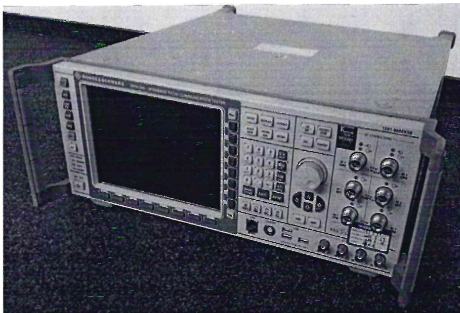
Рисунок 1.1 – Фотография общего вида тестера радиокommunikационного CMW 500 № 151590
