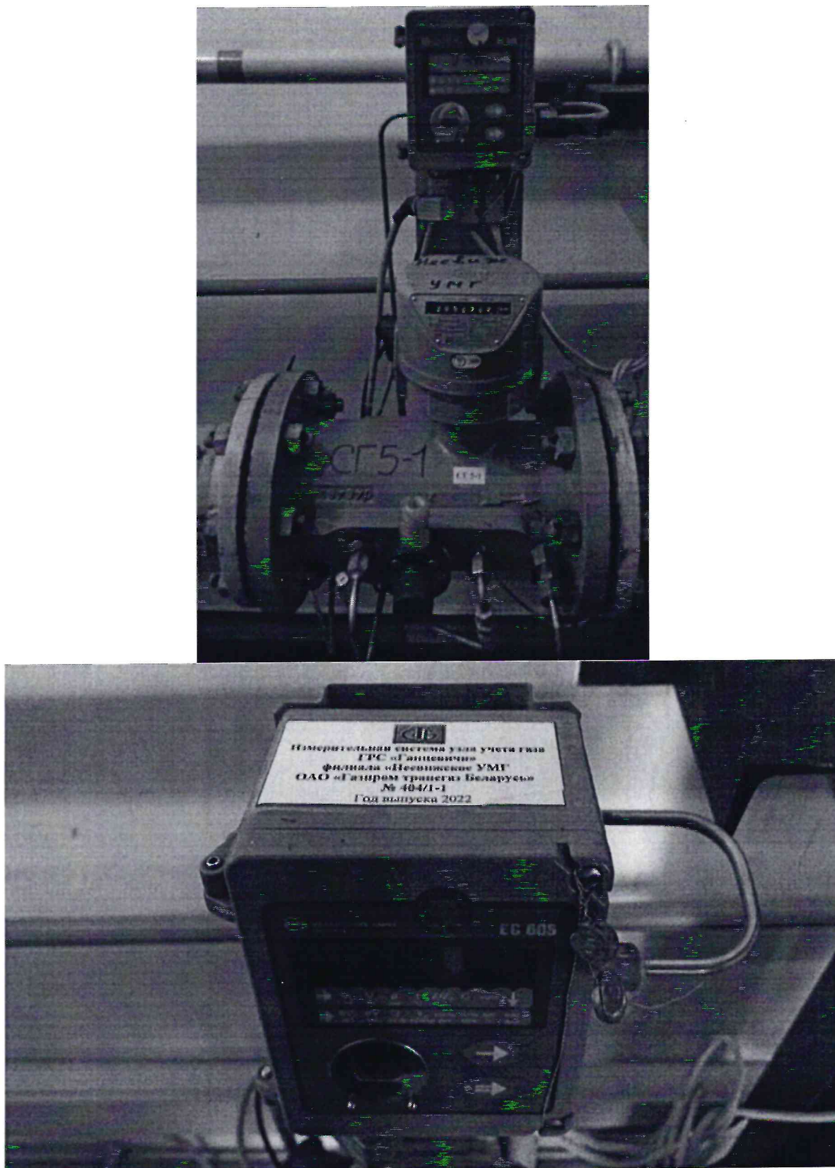
Рисунок 1.1 – Фотографии общего вида ИС УУГ
