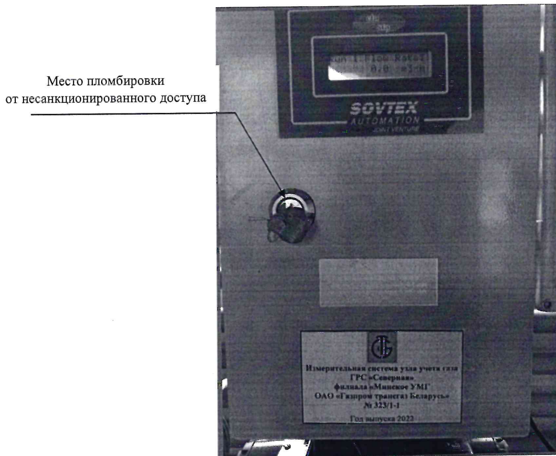
Рисунок 3.1 – Схема пломбировки от несанкционированного доступа
