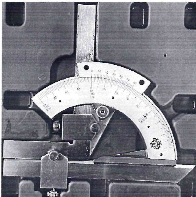
Рисунок 1.1 – Фотография общего вида угломера с нониусом тип 2 № 2403186
