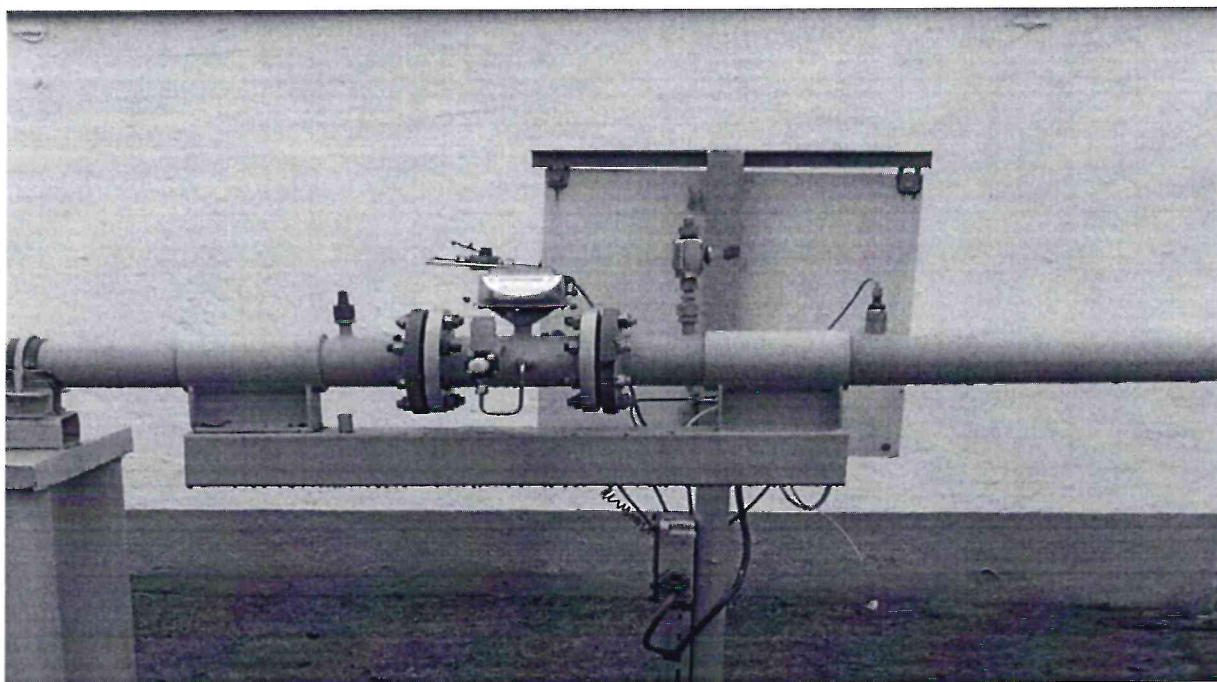
Рисунок 1.1 – Фотографии общего вида ИС УУГ
