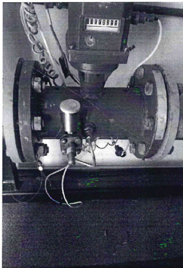
Рисунок 1.1 – Фотографии общего вида ИС УУТ
