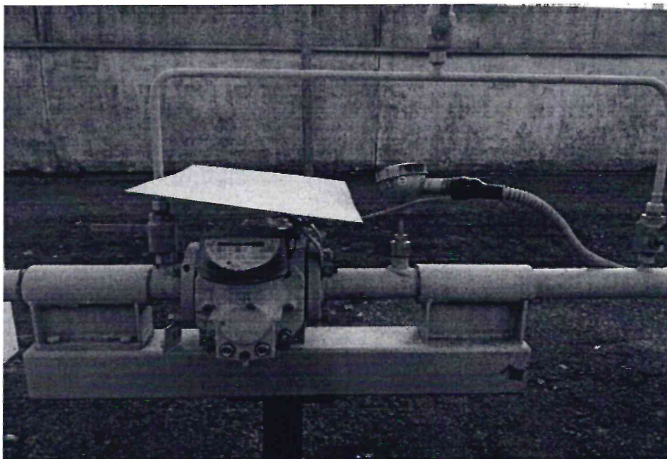
Рисунок 1.1 – Фотография общего вида ИС УУГ
