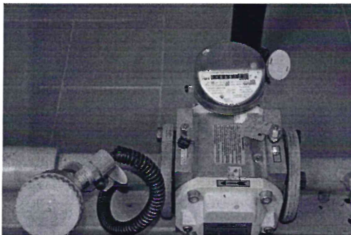
Рисунок 1.1 – Фотографии общего вида ИС УУГ
