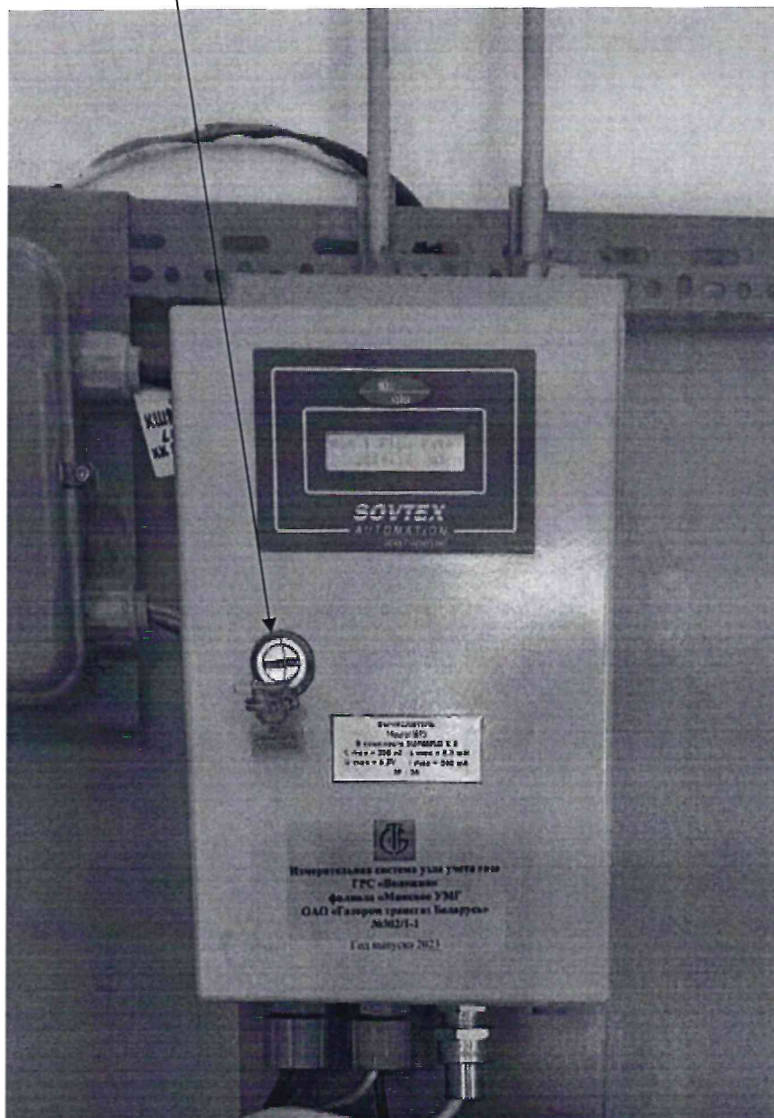
Рисунок 3.1 – Схема пломбировки от несанкционированного доступа
