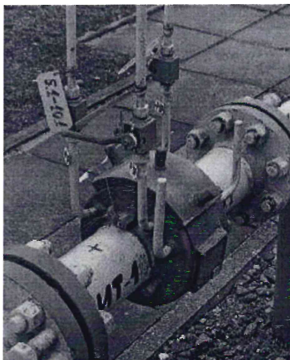
Рисунок 1.1 – Фотографии общего вида ИС УУТ
