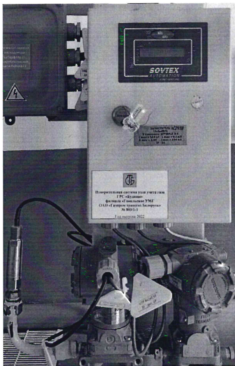
Рисунок 1.1 – Фотографии общего вида ИС УУГ
