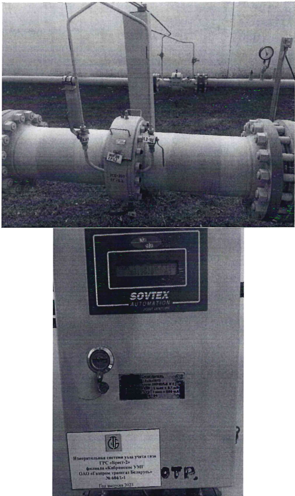
Рисунок 1.1 – Фотографии общего вида ИС УУГ
