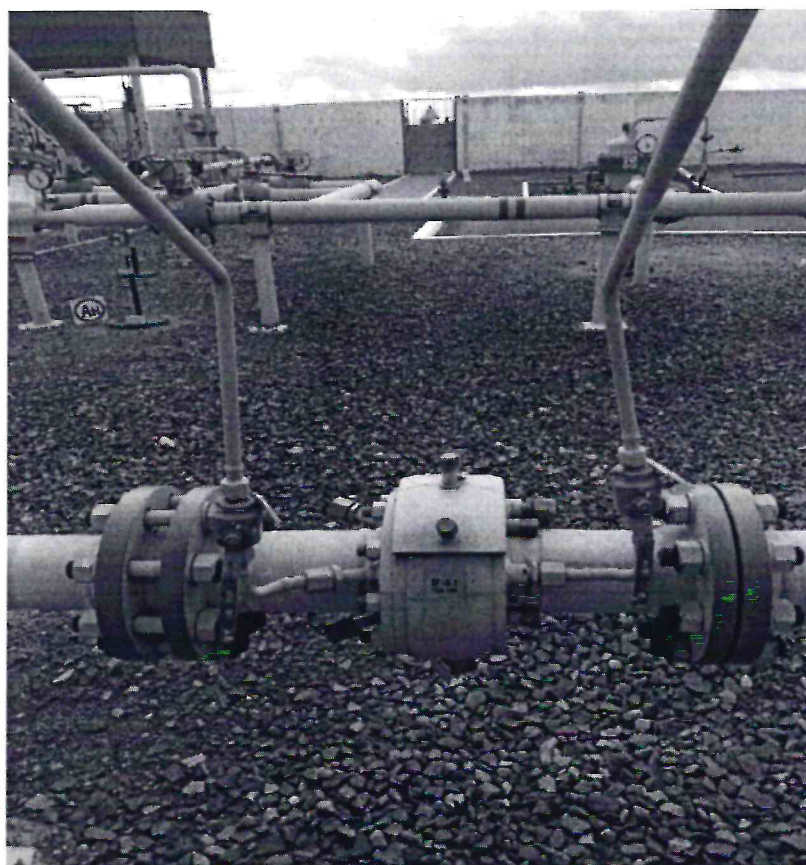
Рисунок 1.1 – Фотографии общего вида ИС УУГ
