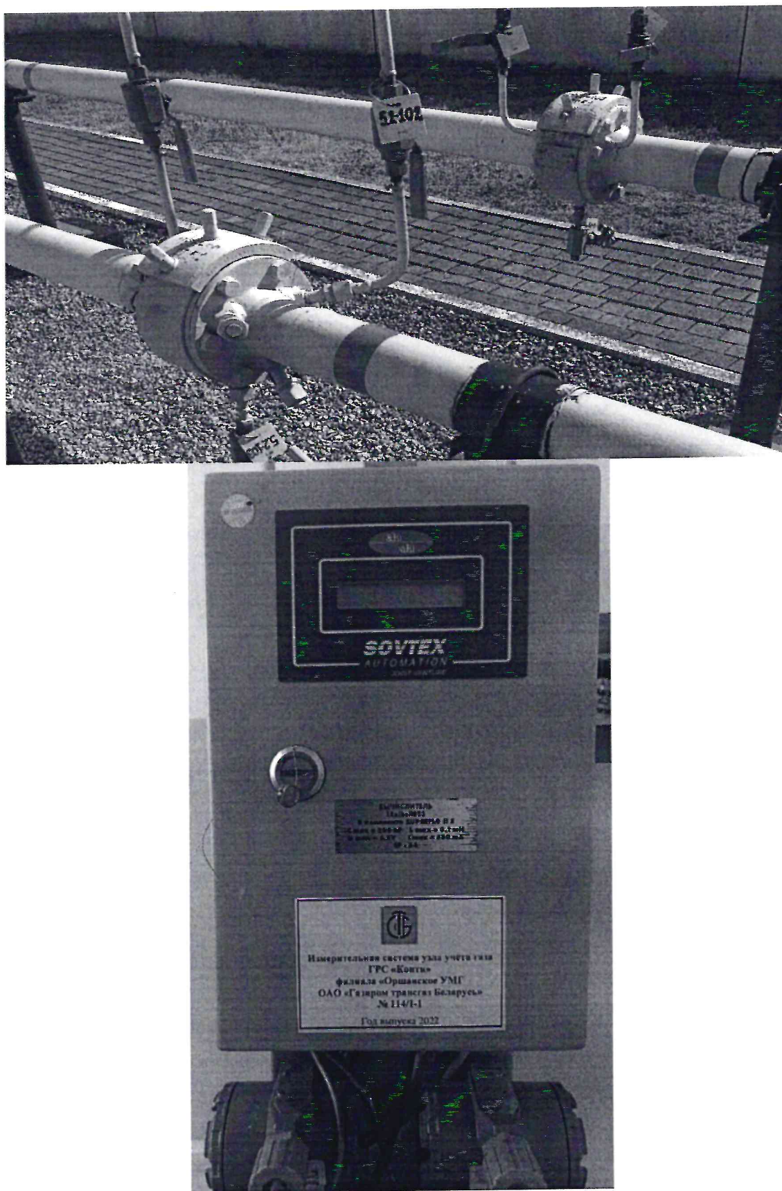
Рисунок 1.1 – Фотографии общего вида ИС УУГ
