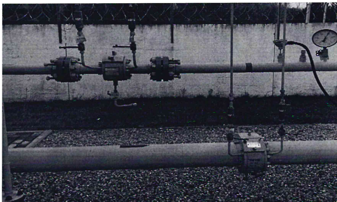
Рисунок 1.1 – Фотографии общего вида ИС УУГ
