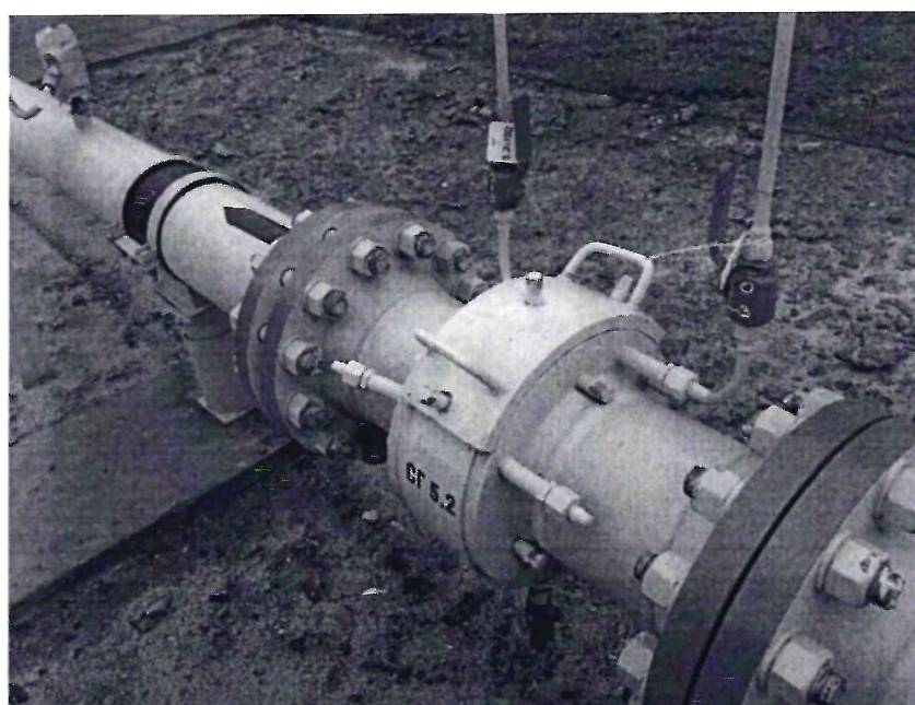
Рисунок 1.1 – Фотографии общего вида ИС УУГ
