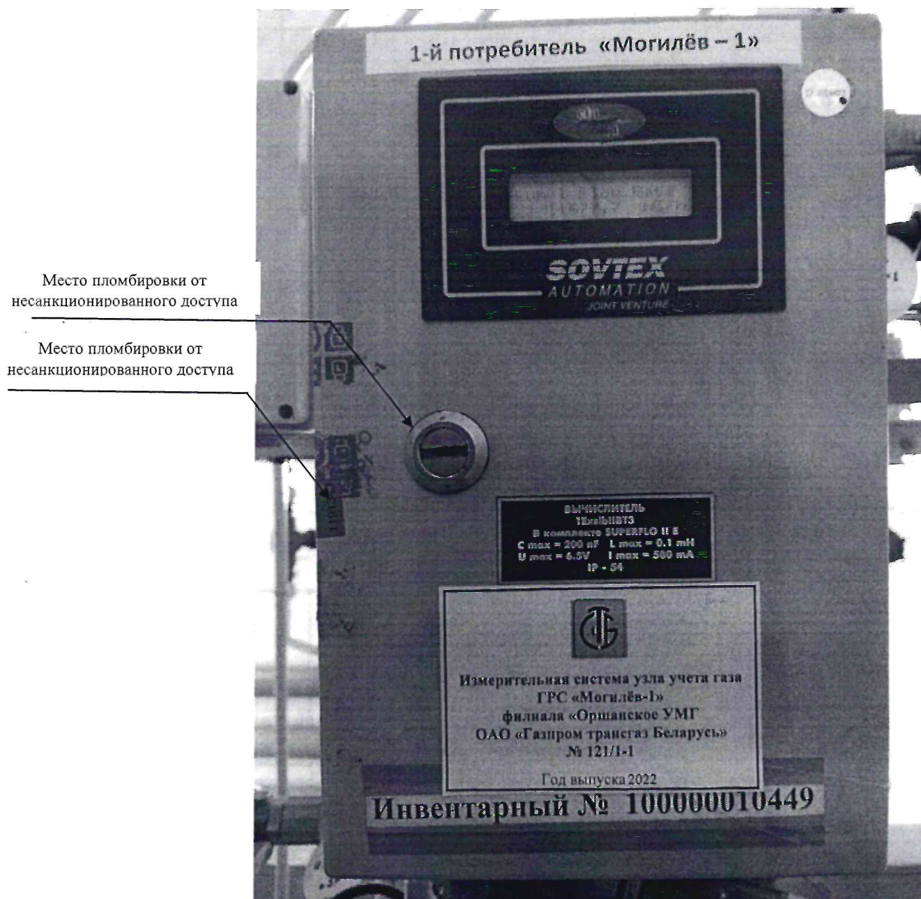
Рисунок 3.1 – Схема пломбировки от несанкционированного доступа
