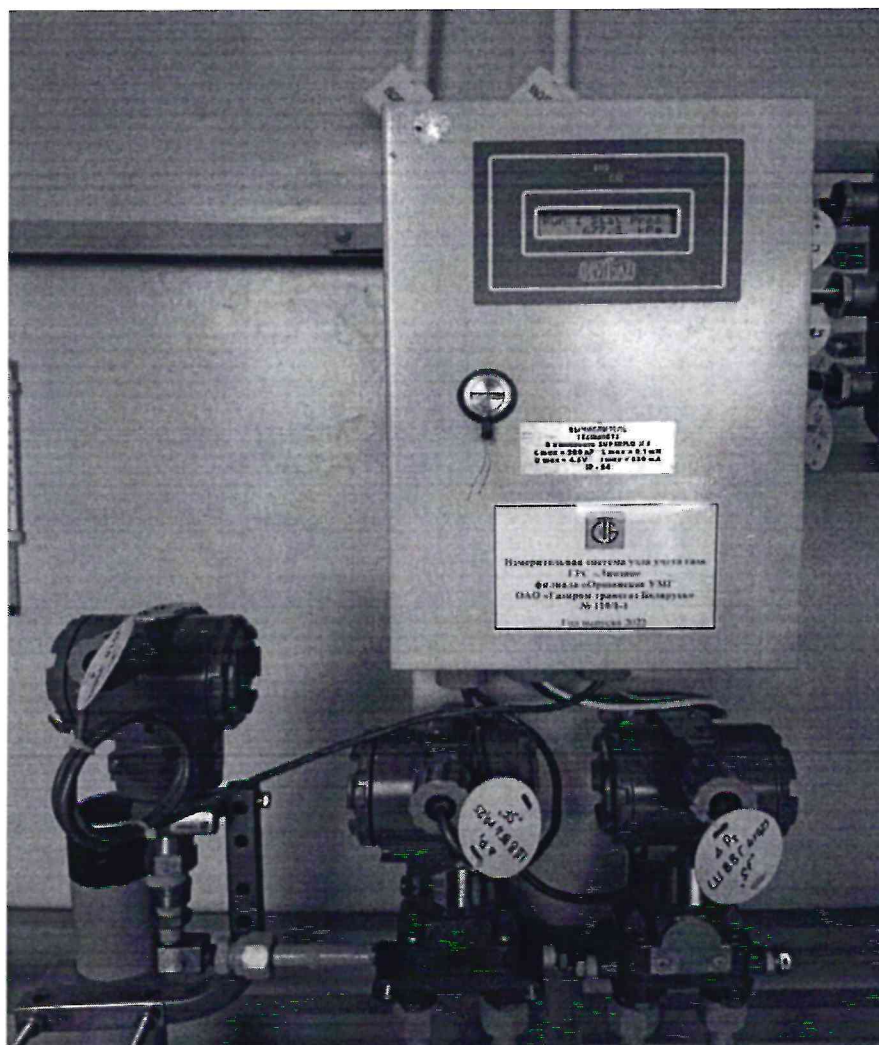
Рисунок 1.1 – Фотографии общего вида ИС УУГ
