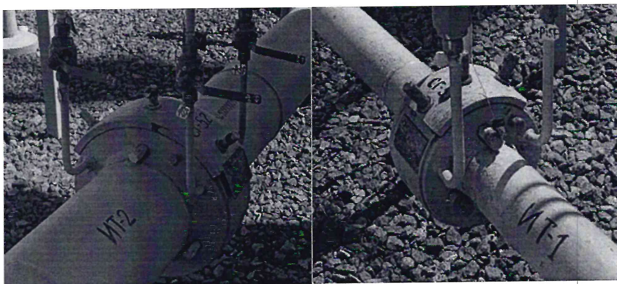
Рисунок 1.1 – Фотографии общего вида ИС УУГ
