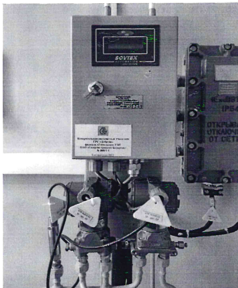
Рисунок 1.1 – Фотографии общего вида ИС УУГ
