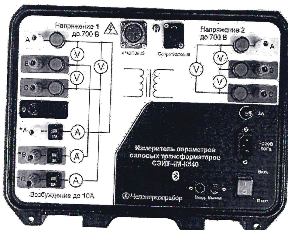
Рисунок 2- Внешний вид ИВБ измерителя СЭИТ-4М-K540 (исполнение 2)
