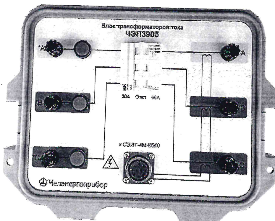
Рисунок 3- Внешний вид БТТ измерителя СЭИТ-4М-K540
