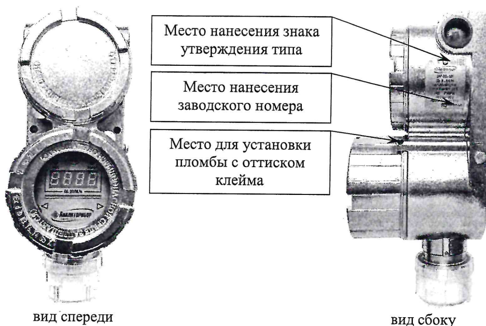
а) в корпусе из нержавеющей стали
