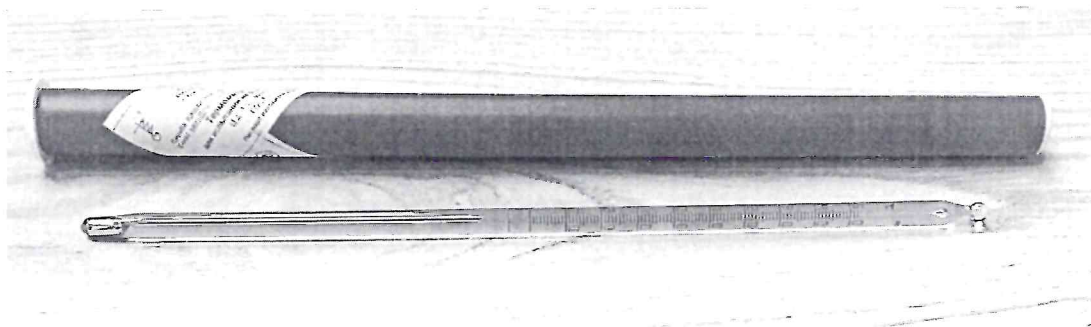
Рисунок 1.1 – Фотография общего вида термометра стеклянного для испытаний нефтепродуктов ТИН 3-1 № 8
