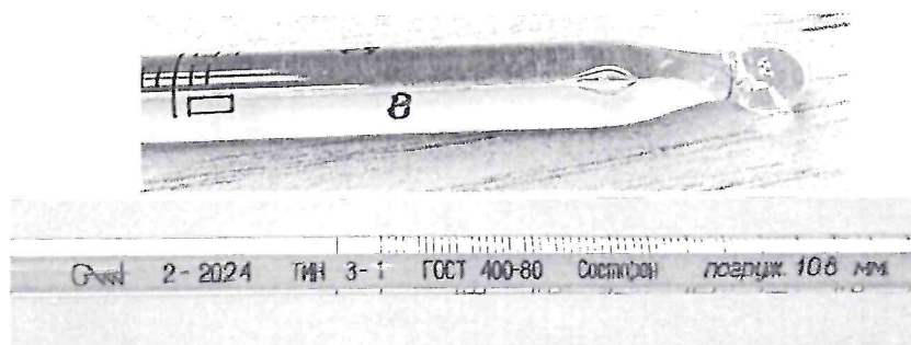
Рисунок 1.2 – Фотографии маркировки термометра стеклянного для испытаний нефтепродуктов ТИН 3-1 № 8
