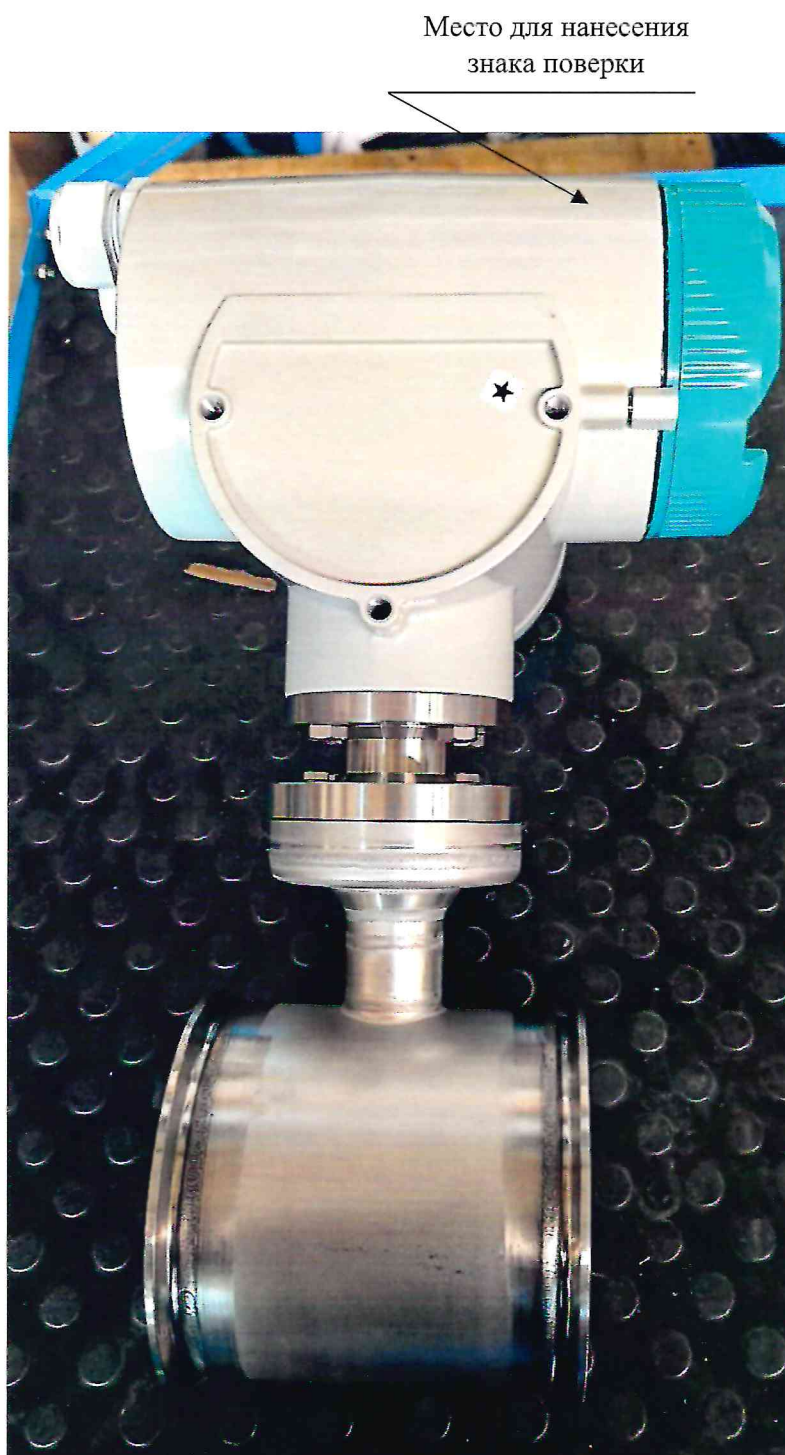
Рисунок 2.1 – Схема (рисунок) с указанием места для нанесения знака поверки
