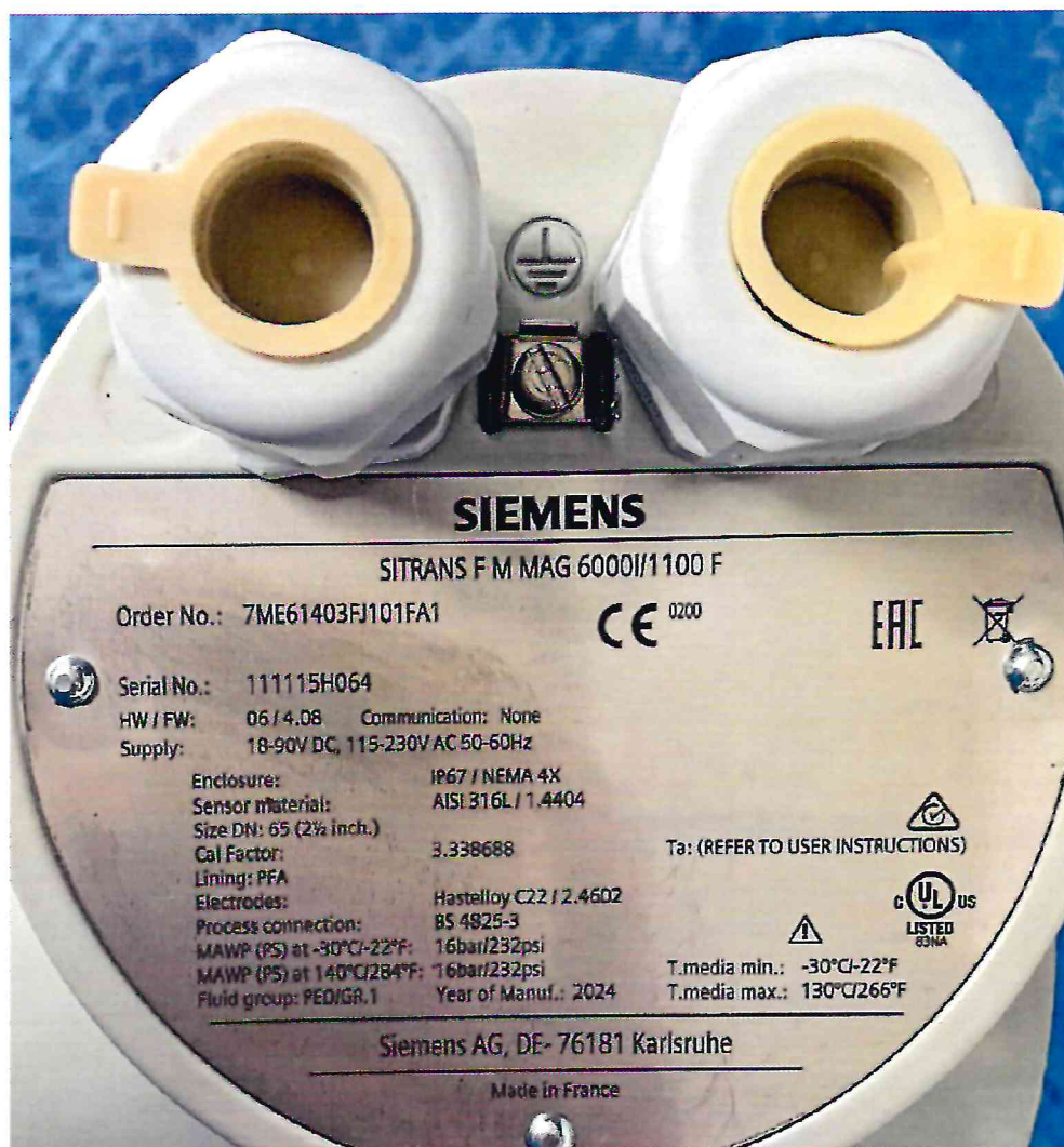
Рисунок 1.2 – Фотография маркировки расходомера-счетчика электромагнитного SITRANS F M MAG 6000I/1100 F № 111115H064
