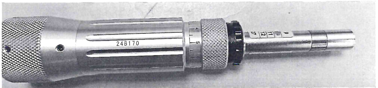
Рисунок 1.2 – Фотография маркировки отвертки динамометрической (моментной) 775/12 № 24B029
