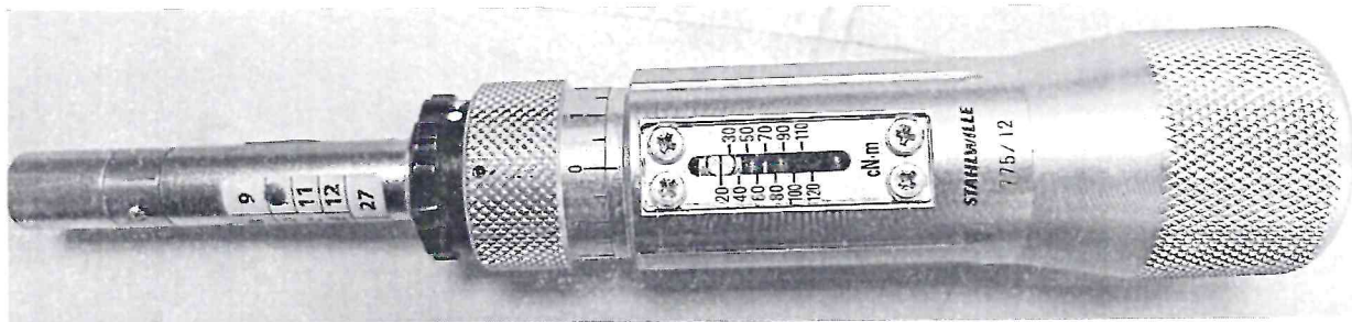
Рисунок 1.1 – Фотографии общего вида отвертки динамометрической (моментной) 775/12 № 24В091
