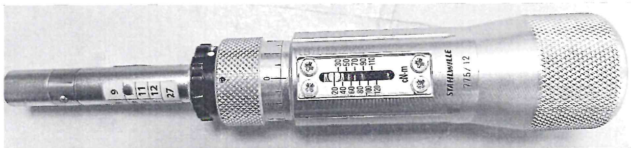
Рисунок 1.1 – Фотографии общего вида отвертки динамометрической (моментной) 775/12 № 24B168
