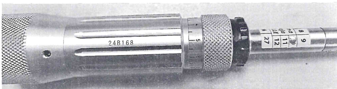
Рисунок 1.2 – Фотография маркировки отвертки динамометрической (моментной) 775/12 № 24B168
