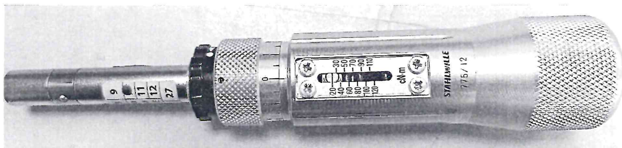
Рисунок 1.1 – Фотографии общего вида отвертки динамометрической (моментной) 775/12 № 24B170
