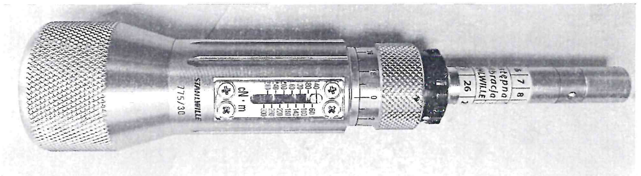
Рисунок 1.1 – Фотографии общего вида отвертки динамометрической (моментной) 775/30 № 231002
