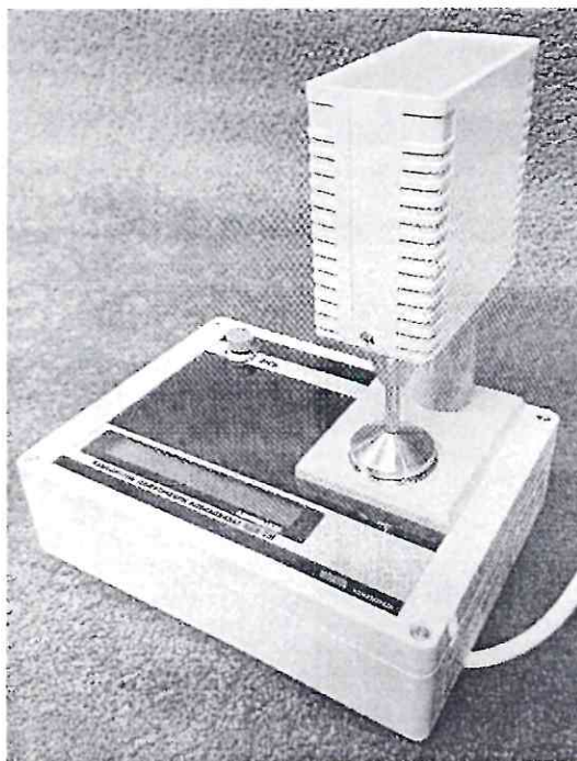
Рисунок 1.1 – Фотография общего вида измерителя деформации клейковины ИДК-ЗМ № 7700
